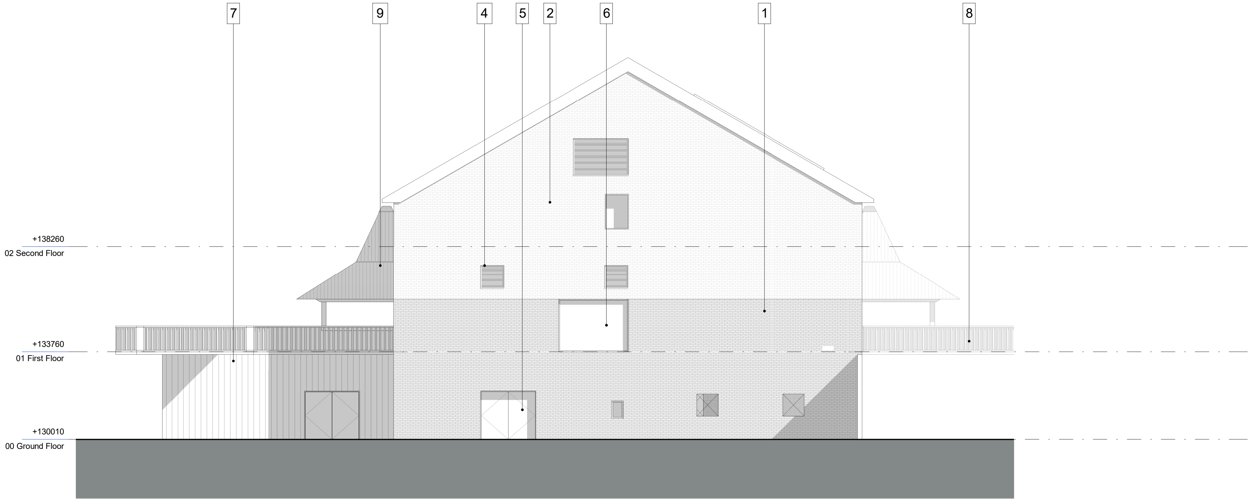
Elevation B: West Scale: 1 : 100
