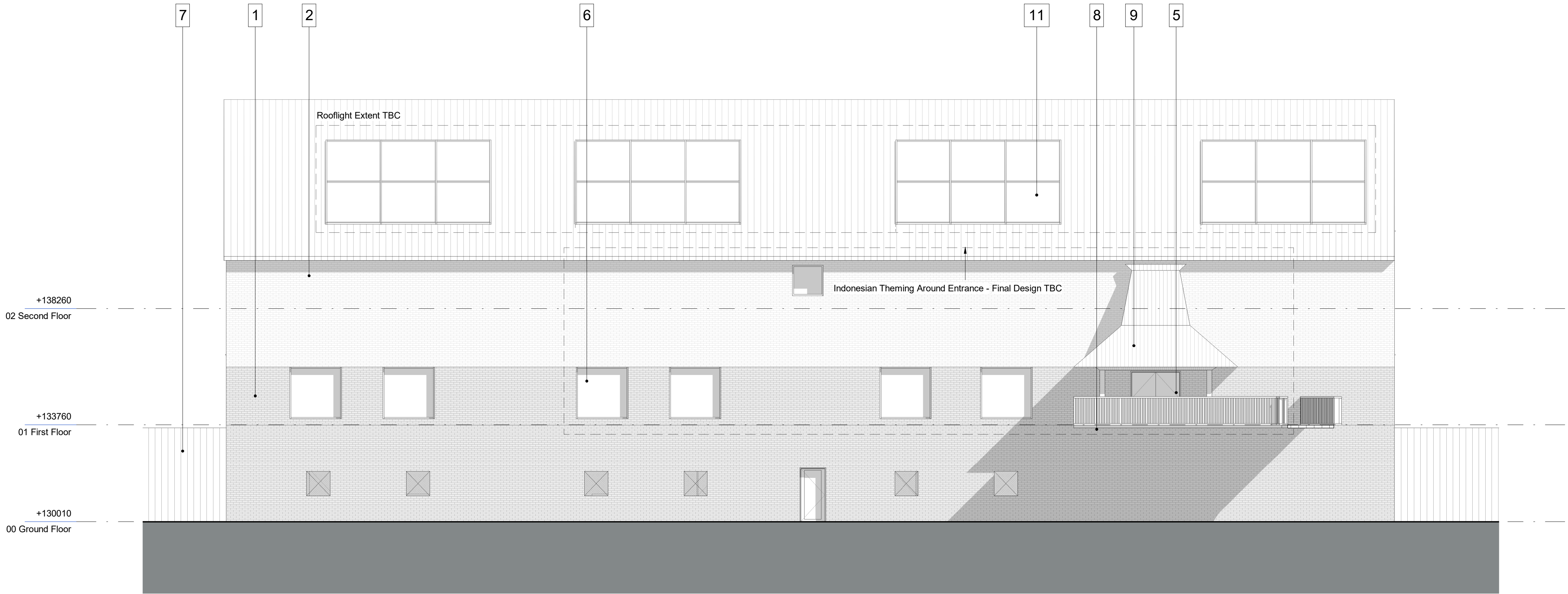
Elevation A: South Scale: 1 : 100
