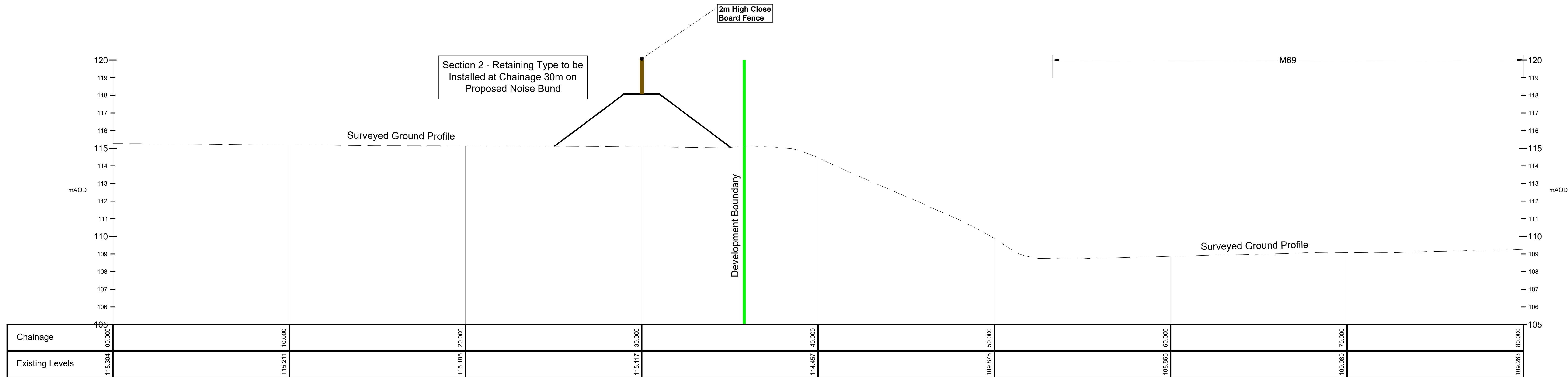
Section B-B Horiz. 1:100, Vert. 1:100
