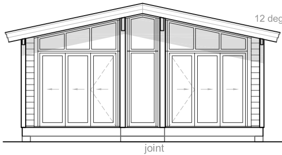
End Elevation
