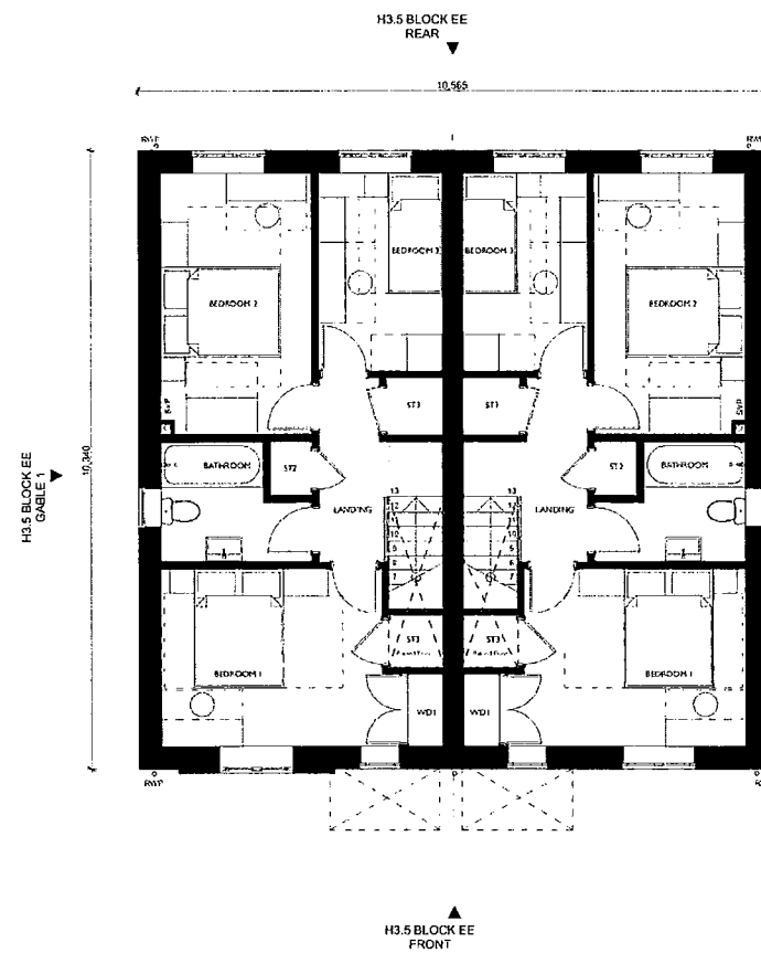
BLOCK E2E FIRST FLOOR 1:100
