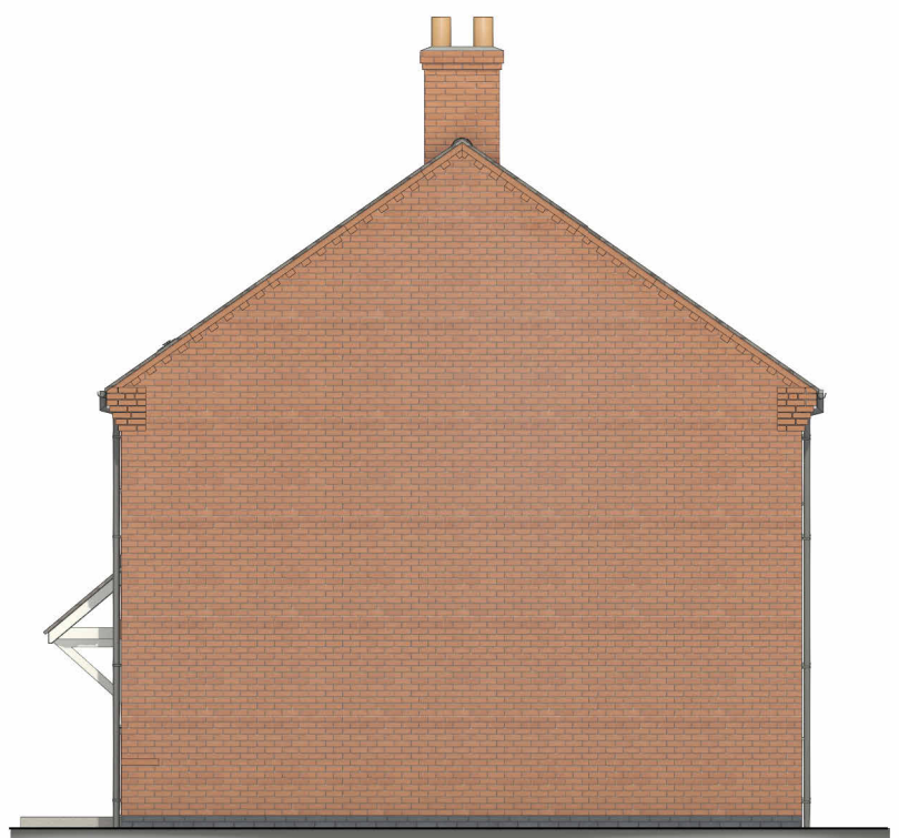
Right Elevation
