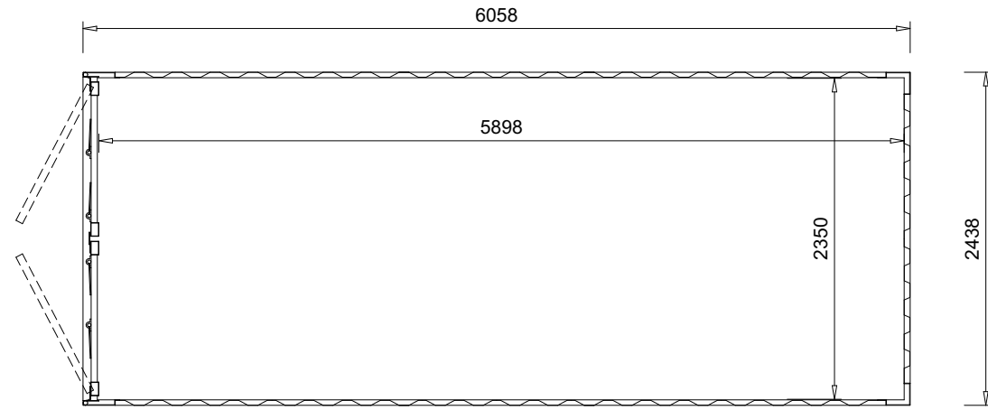
01 CONTAINER PLAN 1:50
