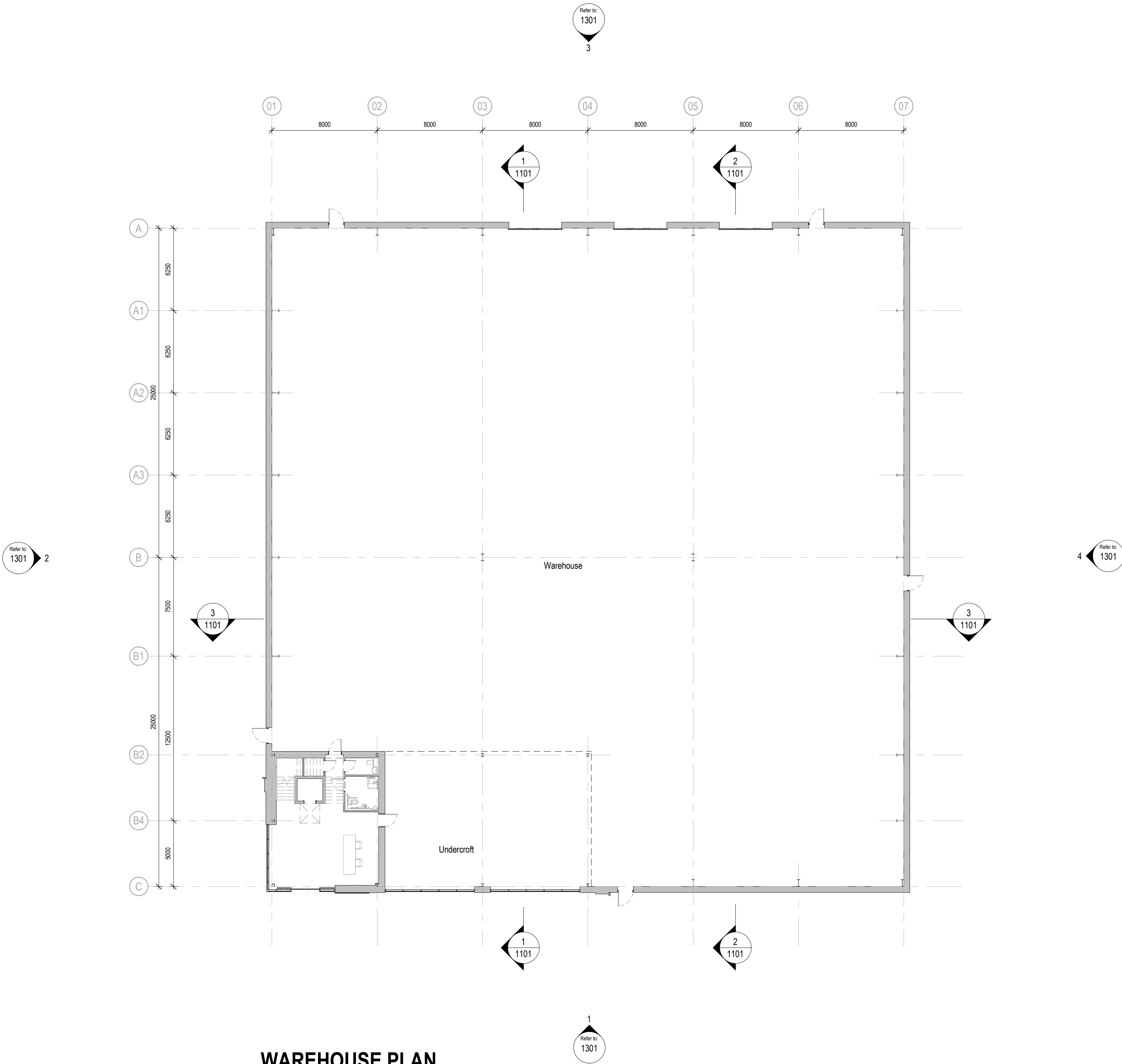
WAREHOUSE PLAN 1 : 200
