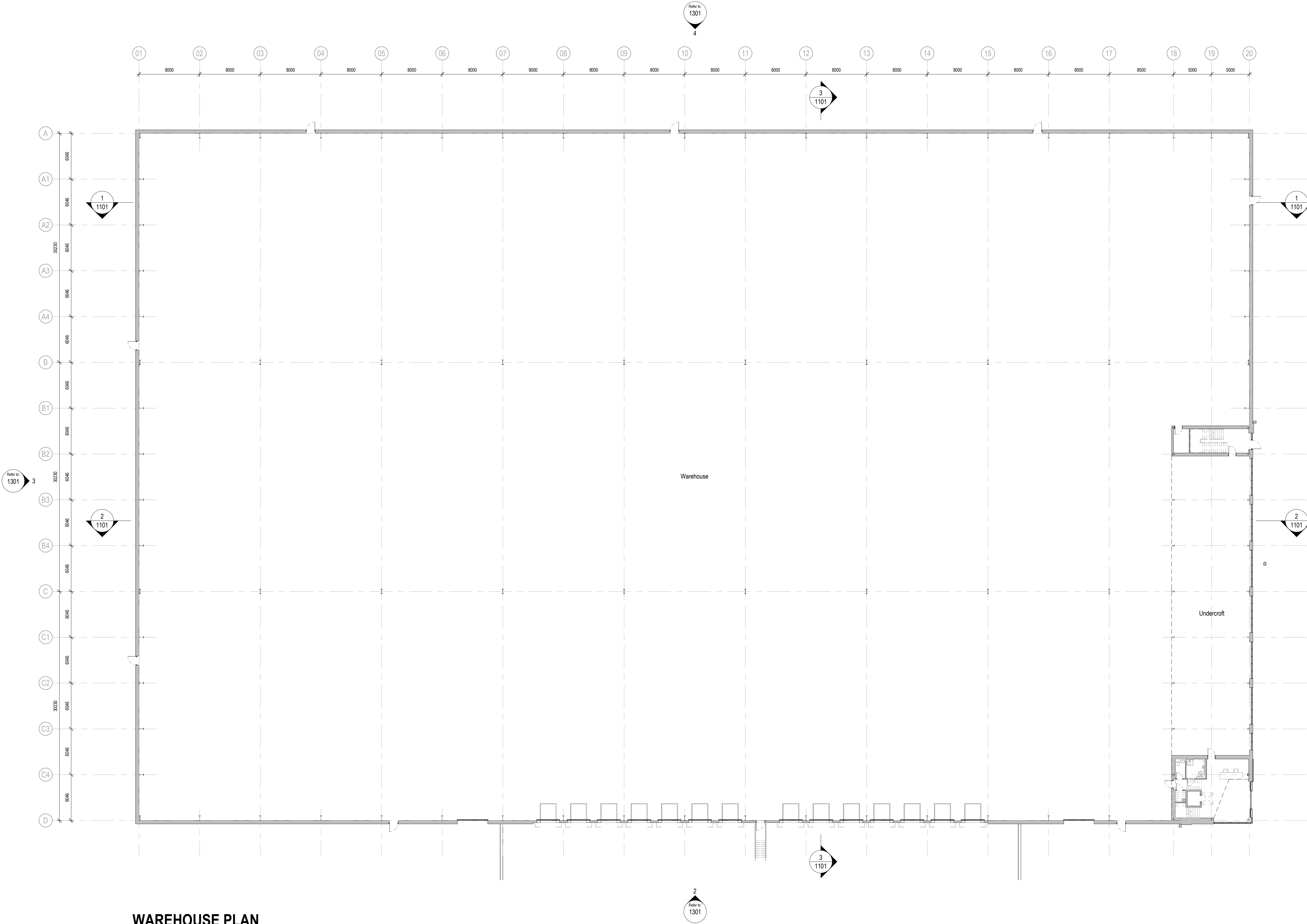
WAREHOUSE PLAN 1 : 250
