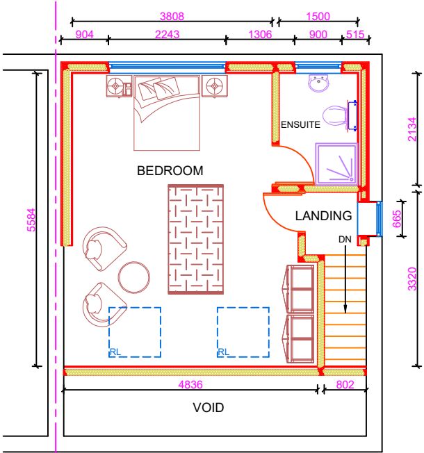
LOFT PLAN
