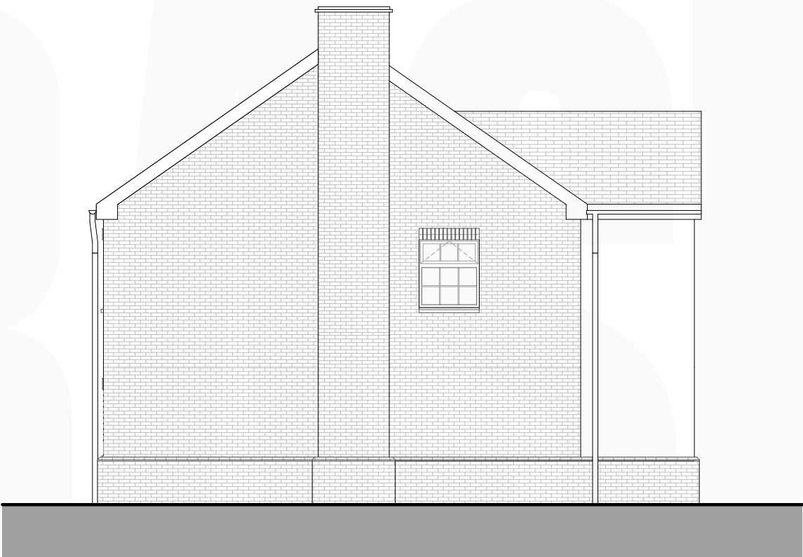
E2 Side Elevation 1:100
