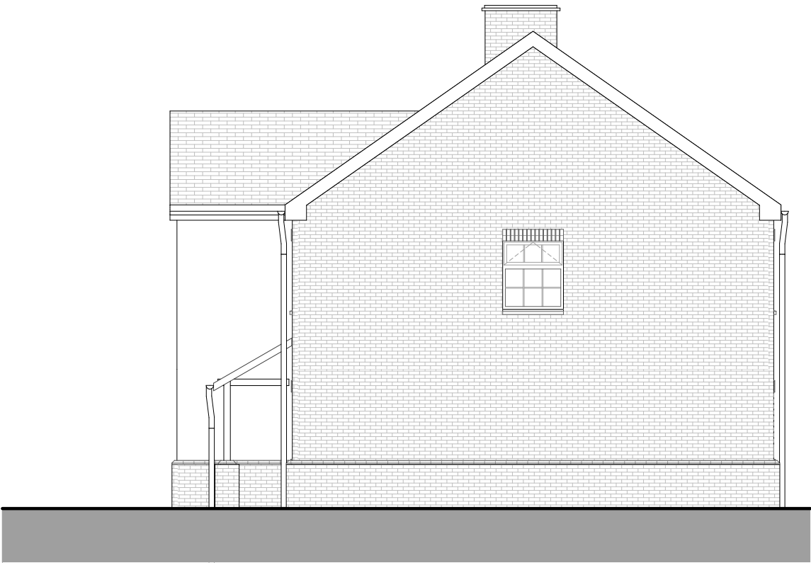
E4 Side Elevation 1:100
