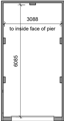
Floor Plan 1 : 100
