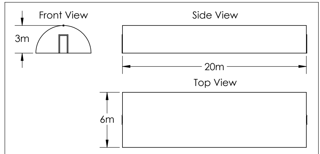
Poly Tunnel Dimensions 1:250
