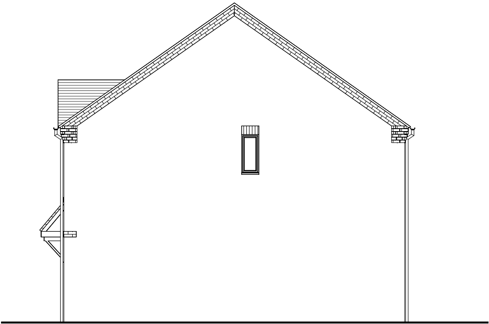
Right Elevation
