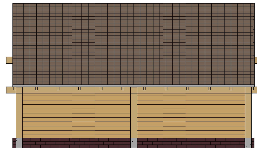
3 West 1 : 50
