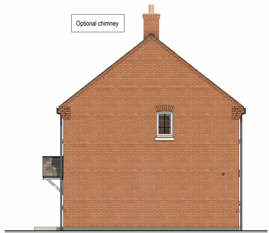
Right Elevation
