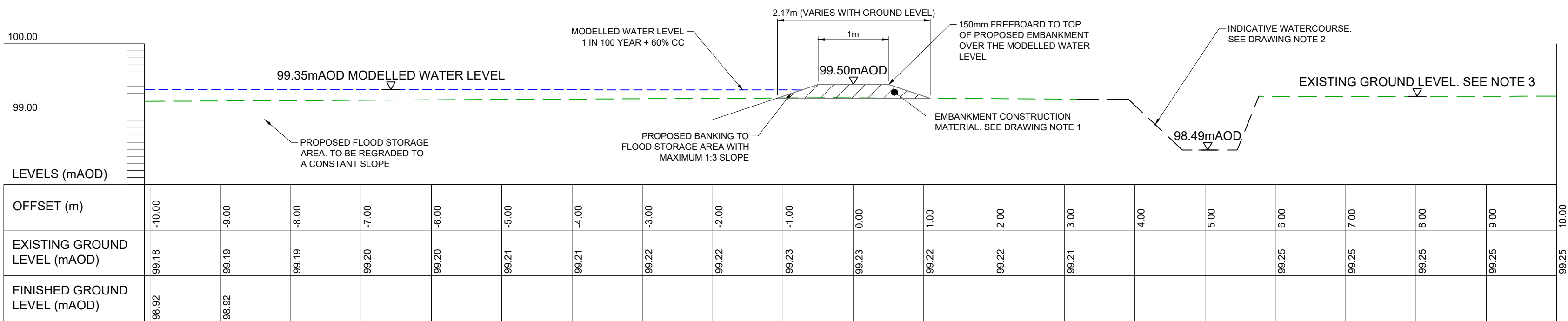
SECTION D-D
