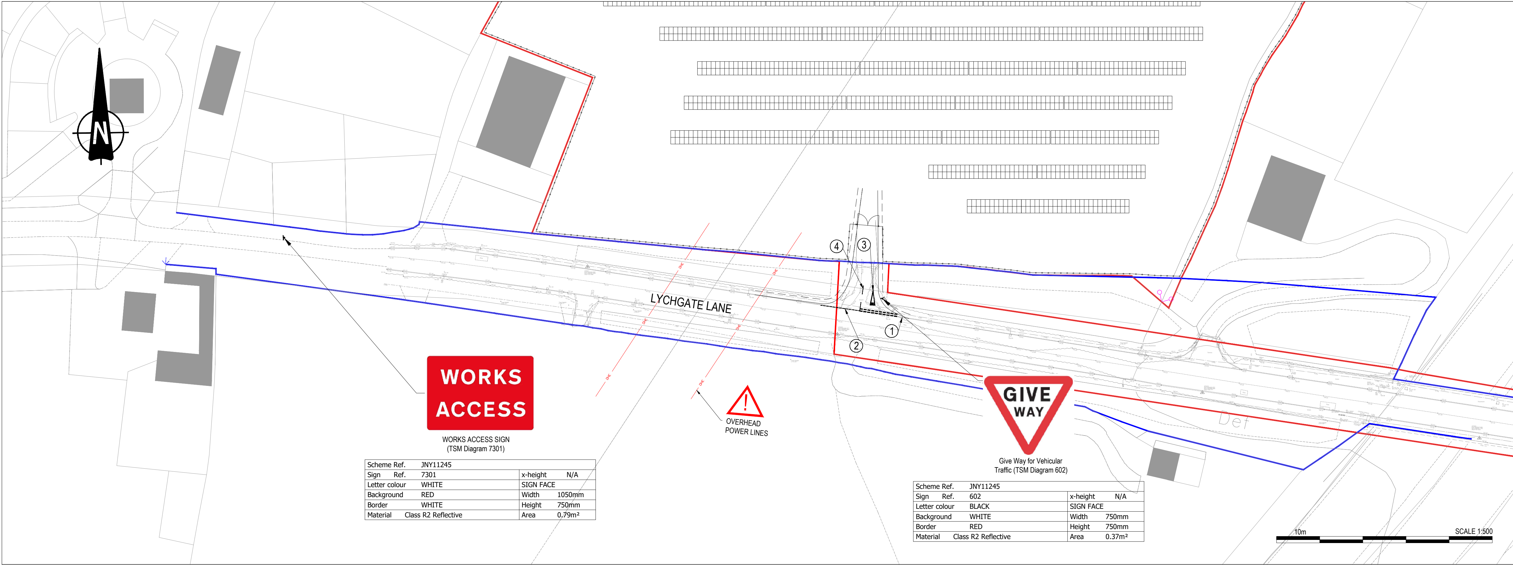
VIEWPORT 1 - PARCEL ACCESS 'A' SCALE: 1:500
