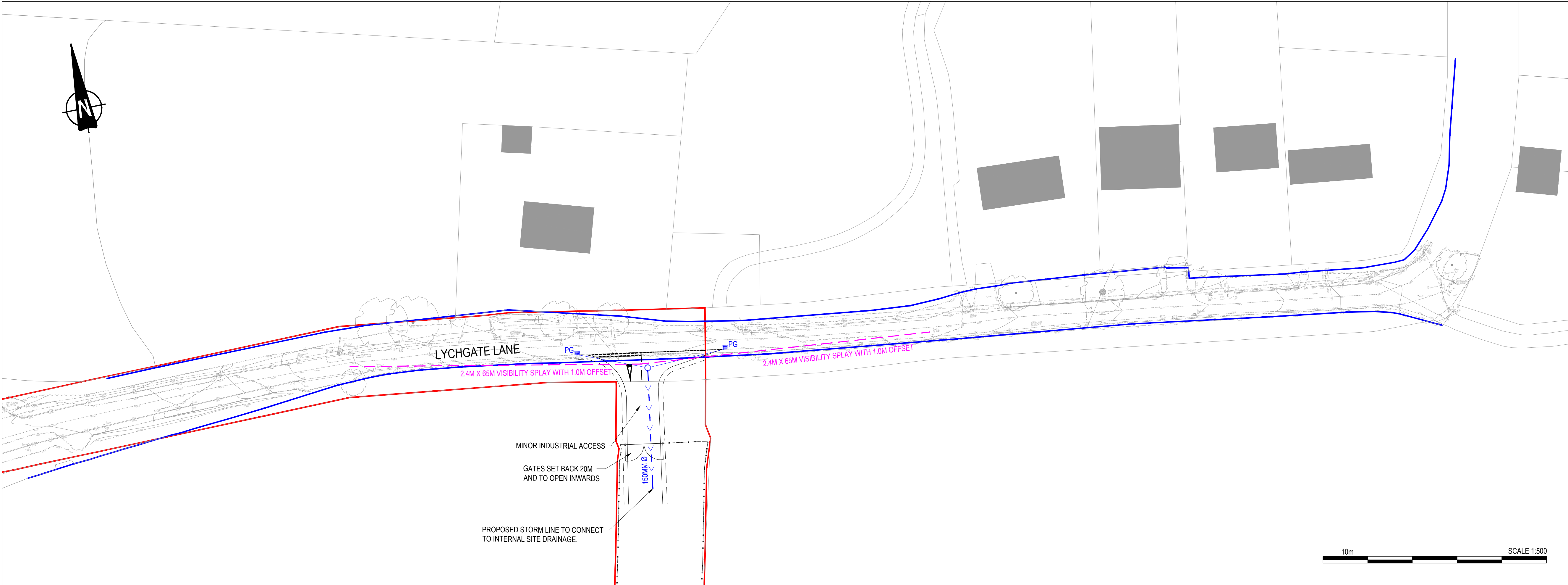
VIEWPORT 2 - PARCEL ACCESS 'B' SCALE: 1:500
