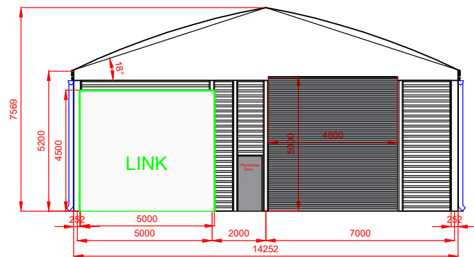
Elevation B
