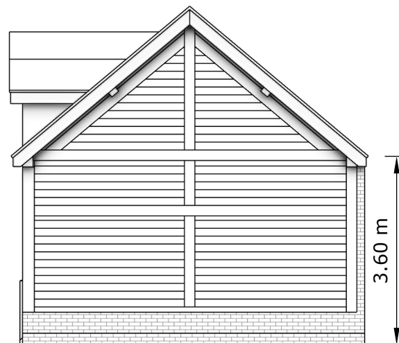
Right Elevation 1:100 @ A3
